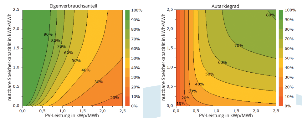
Abbildung 7: Eigenverbrauch in Abhängigkeit von Batterie- und PV-Anlagegrösse, siehe auch www.volker-quaschning.de/artikel/2013-06-Dimensionierung-PV-Speicher/index.php
